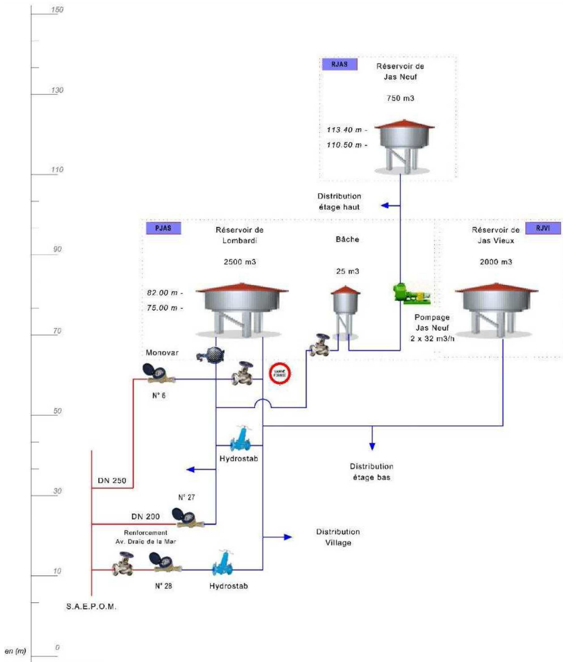
Profil hydraulique des réseaux d’alimentation en eau potable sur Carry-le-Rouet
