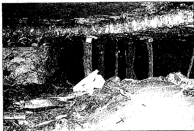
Photo n°2 - Rupture de toit : Guide technique "cavités souterraines"
